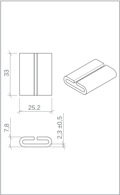
JUNTA CUELQUE
