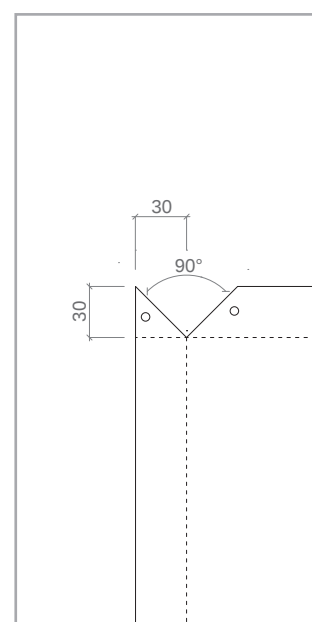
DETALLE B
