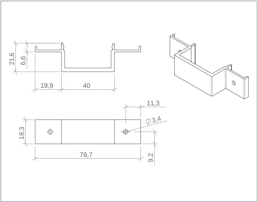
SOPORTE CUELQUE STB-T-CH
