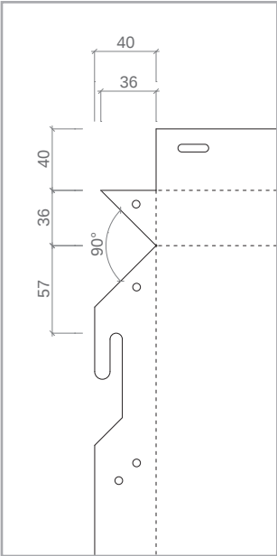
DETALLE B
