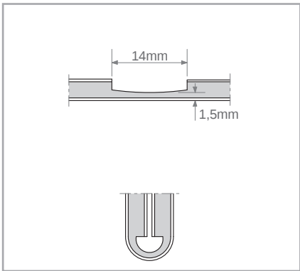
Ranura de fresado en arco para pliegues completos de 180° (no realizable en panel STACBOND® A2 ).
