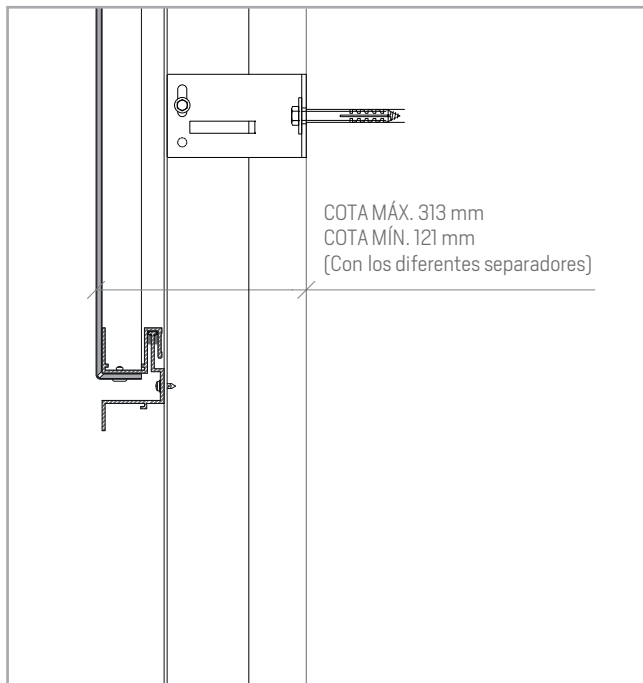
SECCIÓN VERTICAL
