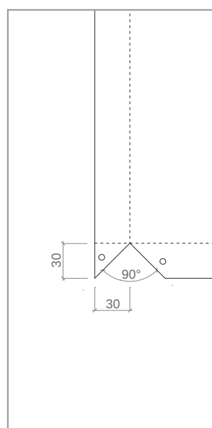
DETALLE A
